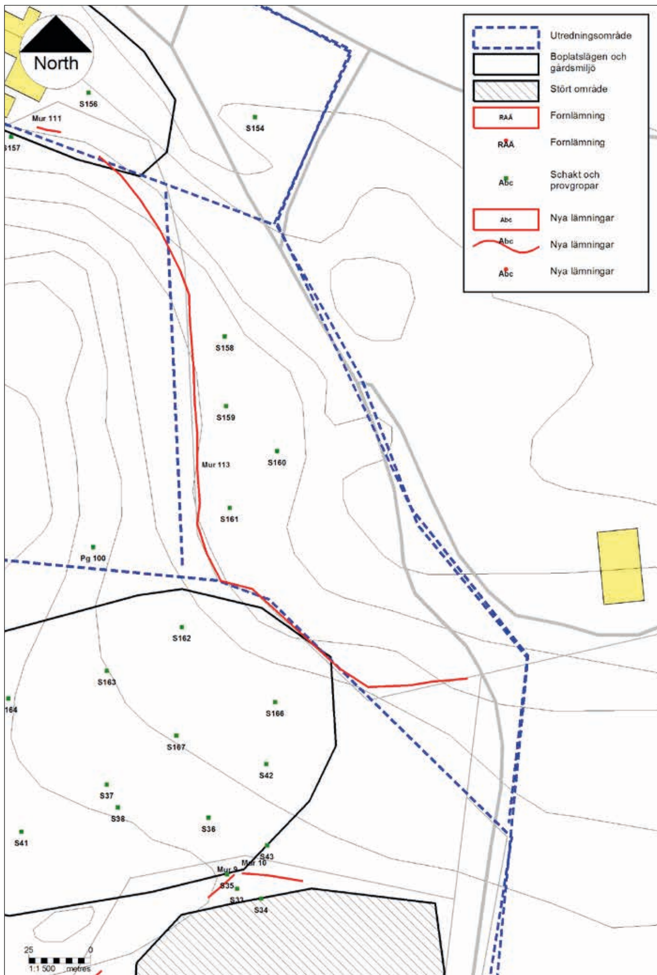
Figur 26. Översiktskarta över Tillägsområde 1 med schakt och dokumenterade gårdesgårdar. Skala 1:500.
