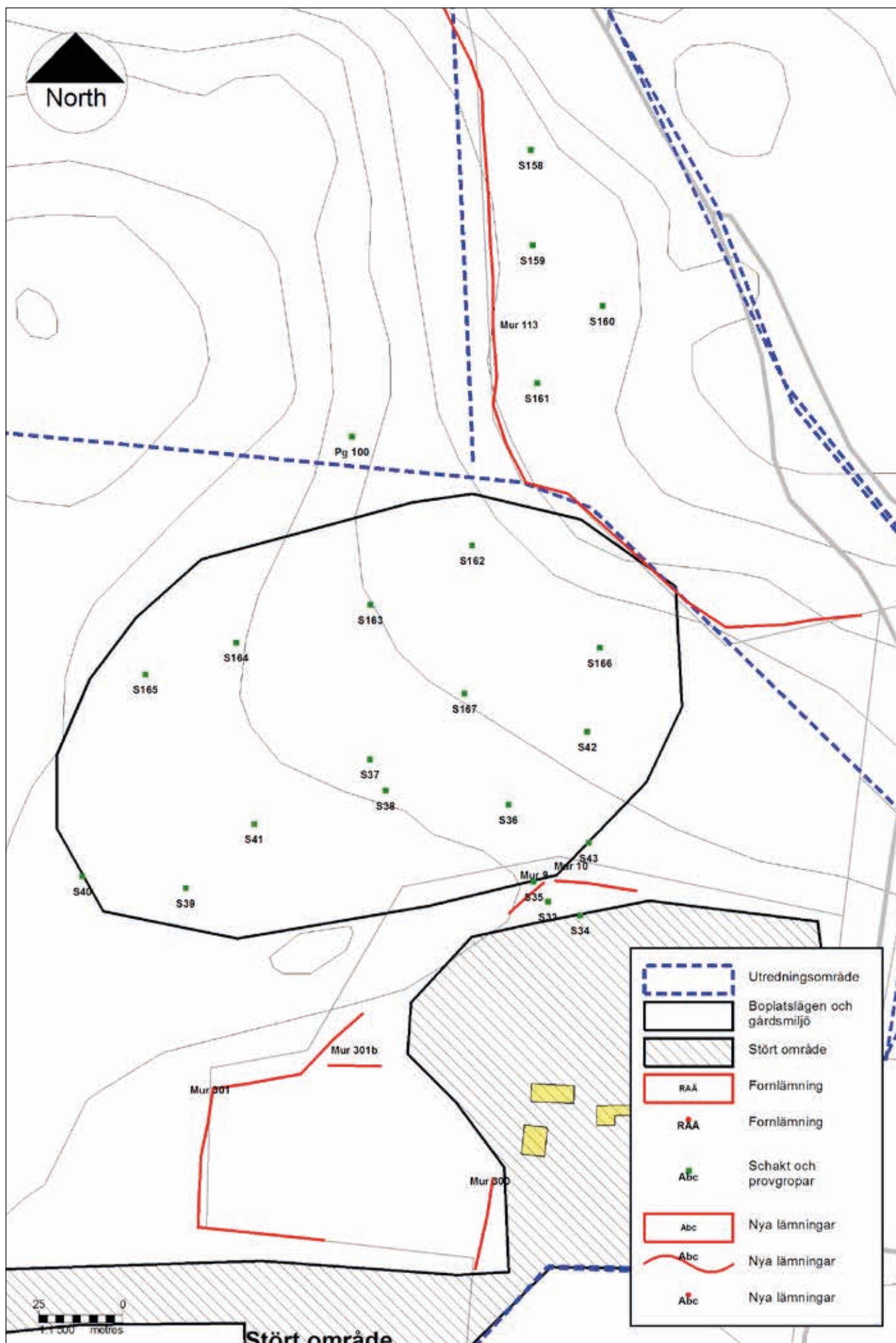
Figur 20. Översiktskarta över Boplatsläge 4 med schakt, provgropar och dokumenterade gårdesgårdar. Skala 1:1 500.
