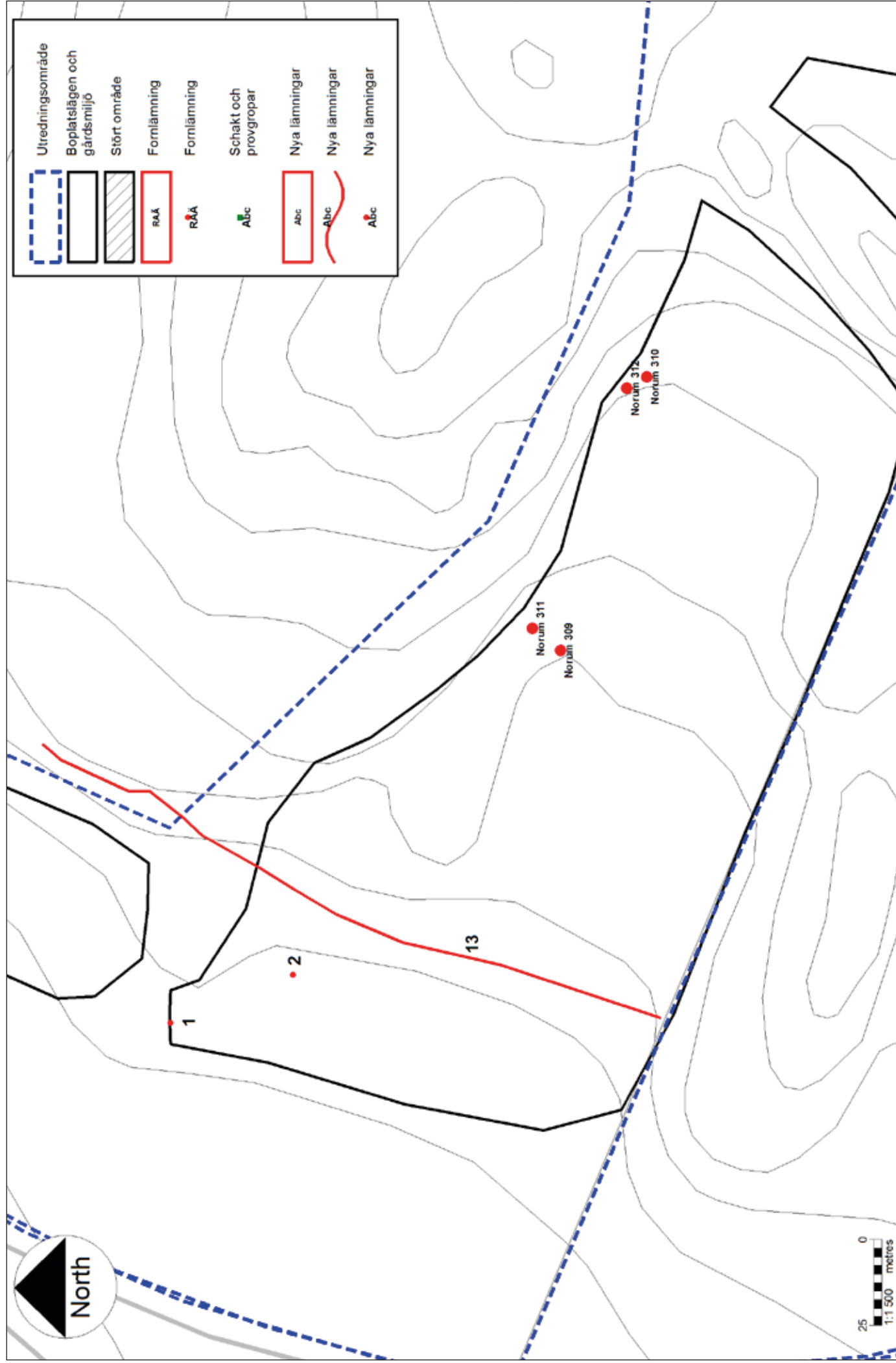
Figur 39. Översiktskarta över Boplatsläge 2 med två nya fornlämningar (1-2) och en övriga kulturhistorisk lämning (13). Med på kartan är också de tidigare kända fornlämningarna Norum 309-312. Skala 1:1 500.
