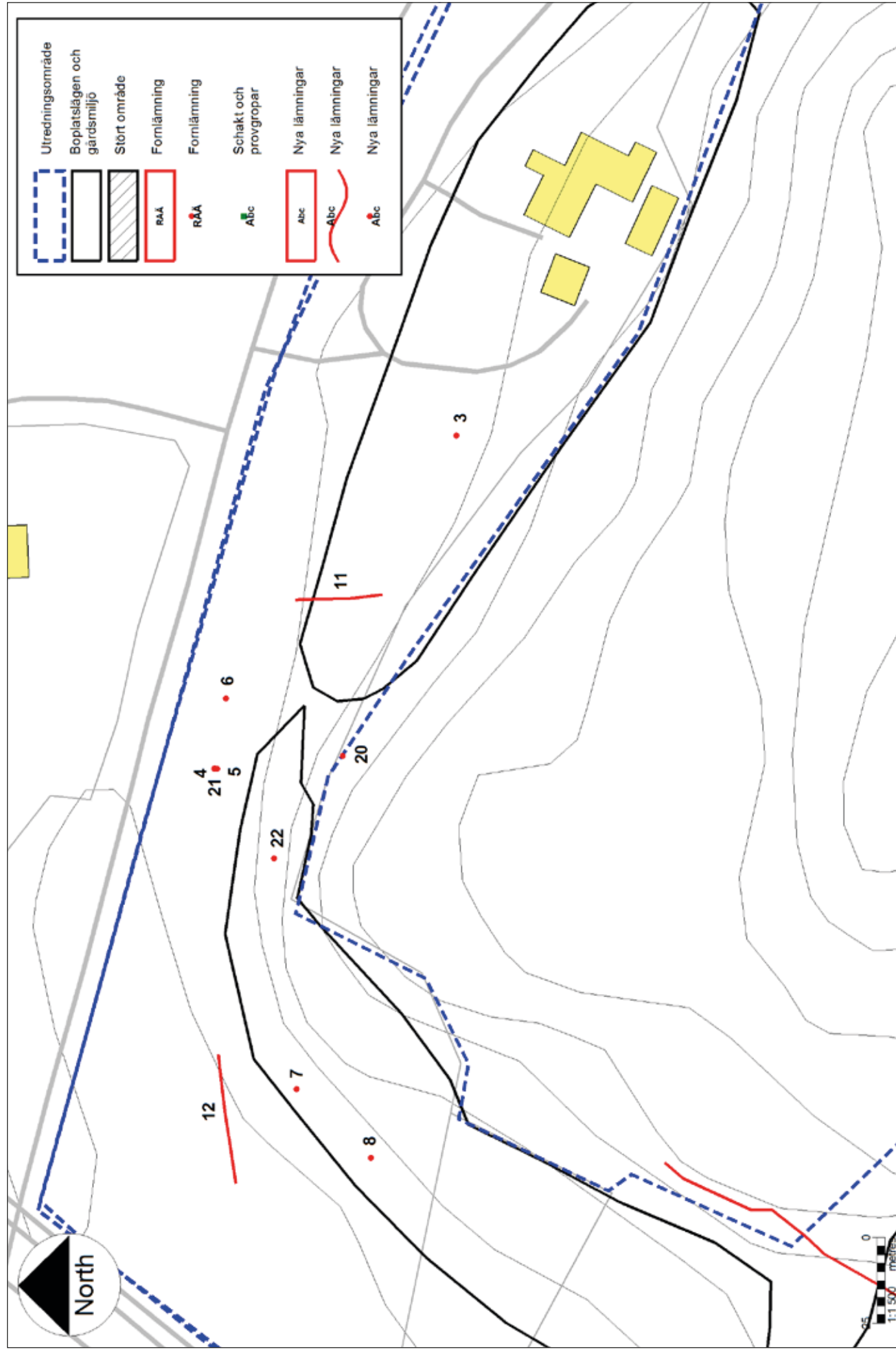
Figur 33. Översiktskarta över Boplatssläge 1 samt Kärr Gårdsmiljö med fyra nya fornlämningar (4-7) och fem övriga kulturhistoriska lämningar (11-12; 20-22). Skala 1:1500.
