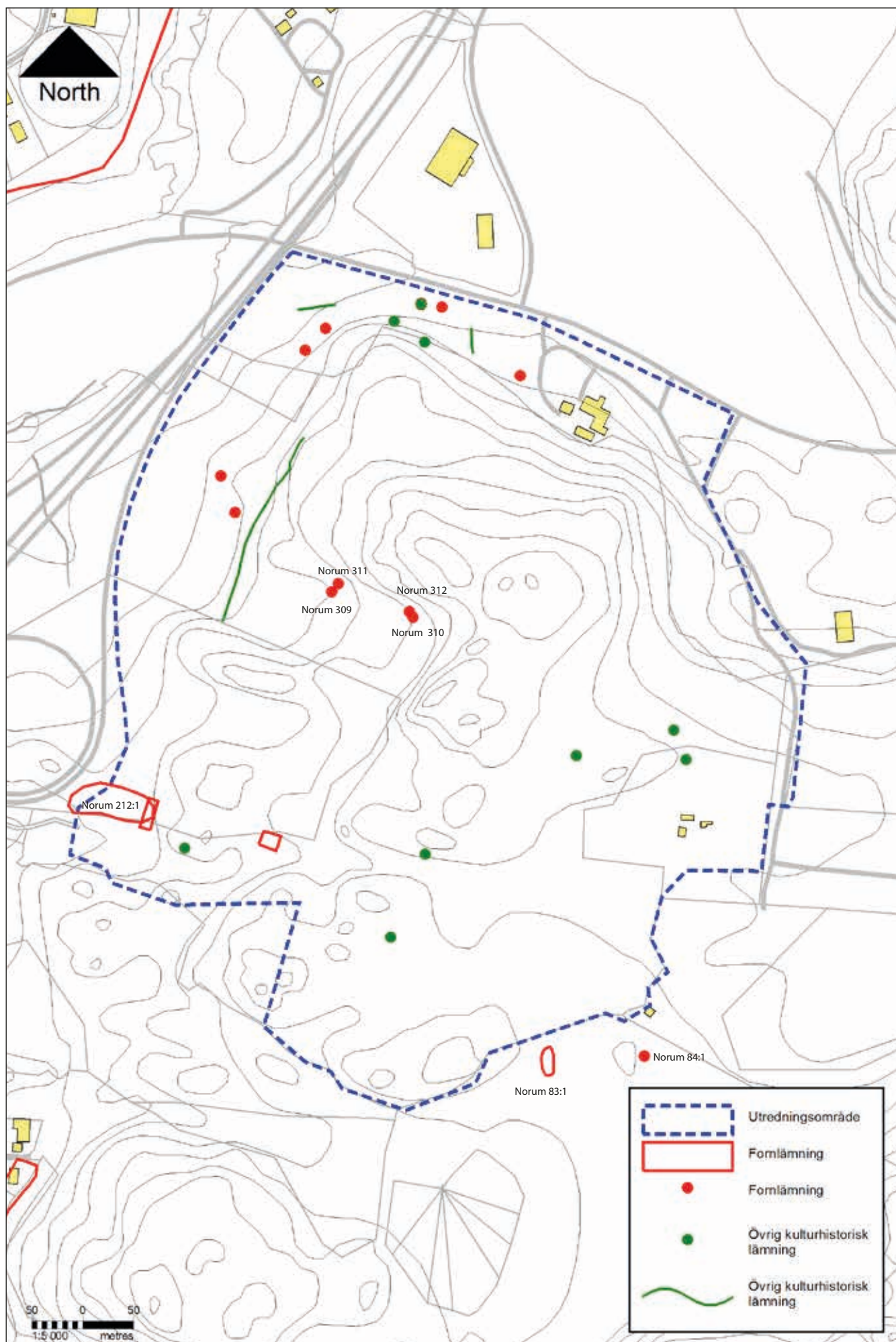
Figur 48. Översiktskarta över hela utredningsområdet med tidigare kända fornlämningar (med RAÄ-nr) samt nya fornlämningar och övriga kulturhistoriska lämningar utmarkerade. Skala 1: 5000.
