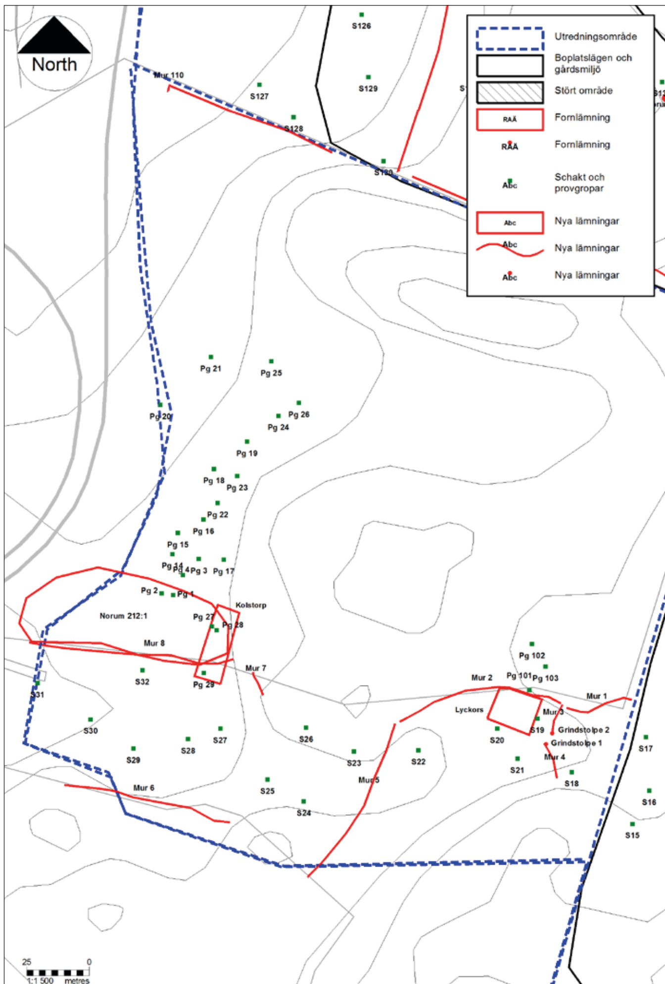
Figur 30. Översiktskarta över Tilläggssområde 2 med schakt, provgropar, dokumenterade gärdesgårdar, grindstolpar och husgrunder. Skala 1:500.
