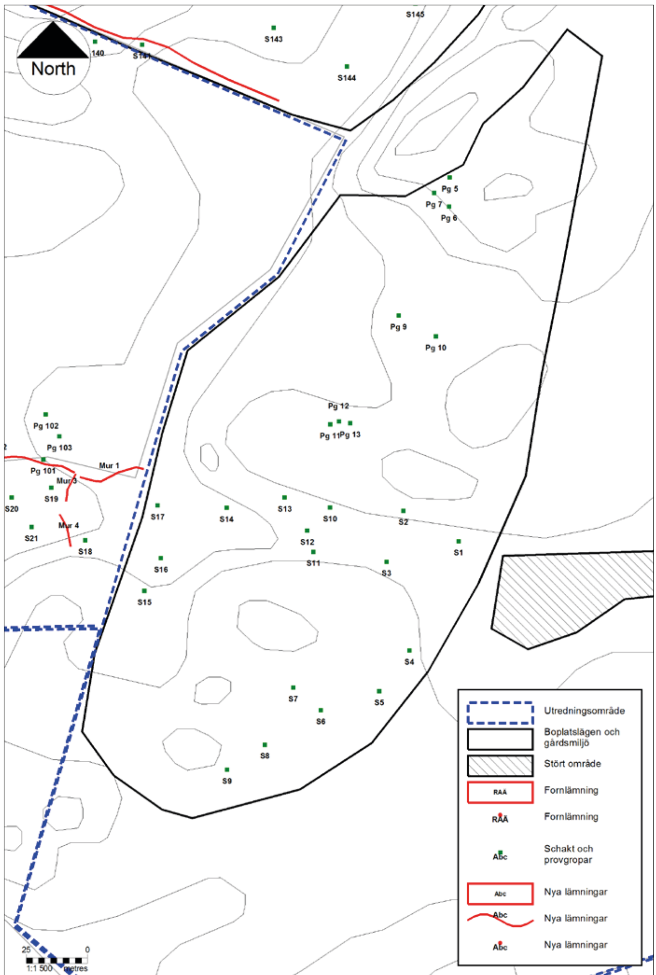
Figur 16. Översiktskarta över Boplatsläge 3 med schakt och provgropar. Skala 1:1 500.
