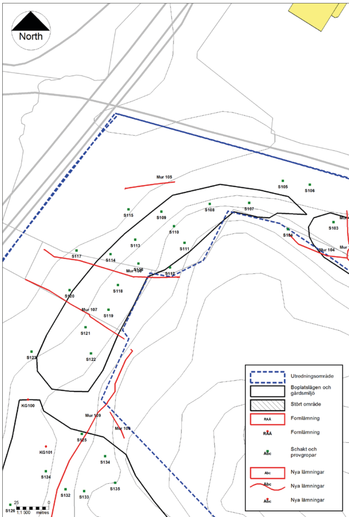
Figur 9. Översiktskarta över Boplatssläge 1 med schakt och och dokumenterade gårdesgårdar. Skala 1:1500.
