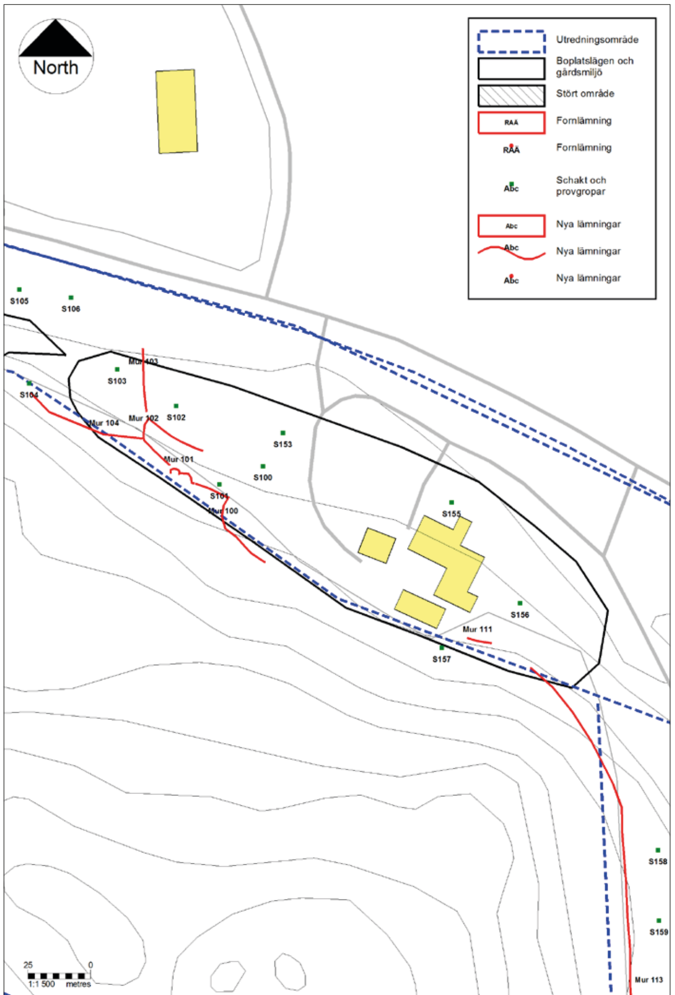
Figur 23. Översiktskarta över Kärr Gårdsmiljö med schakt och dokumenterade gårdesgårdar. Skala 1:1 500.
