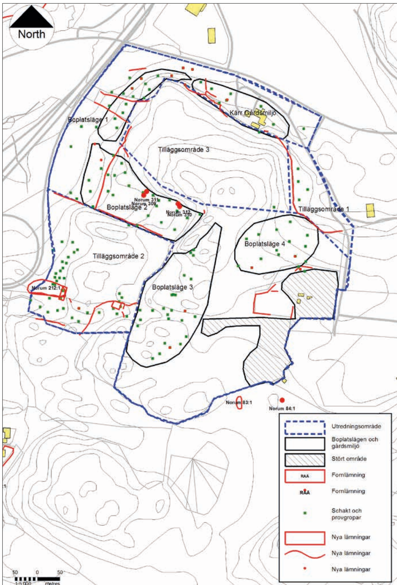
Figur 2. Översiktskarta över utredningsområdet med de fyra olika boplatslägena aktuella för utredning steg 2 samt de tre tilläggsområdena aktuella för steg 1-2 utmarkerade. Tidigare kända fornlämningar är markerade i rött med tillhörande RAÄ-nr medan nya fornlämningar och övriga kulturhistoriska lämningar är markerade endast i rött. Skala 1:5000
